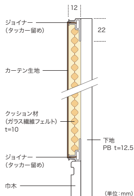
＜ファブリックウォールの構造＞
